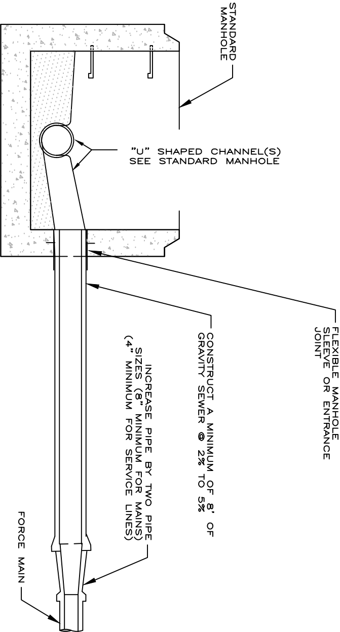
SECTION F—F
